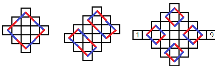
5.4. ábra. Az alternáló körrendszerek
