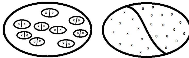
7.1. ábra. Párosítások és színezések
