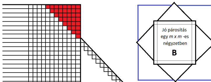
5.8. ábra. Egy anomáliamentes párosítás kiterjedése
