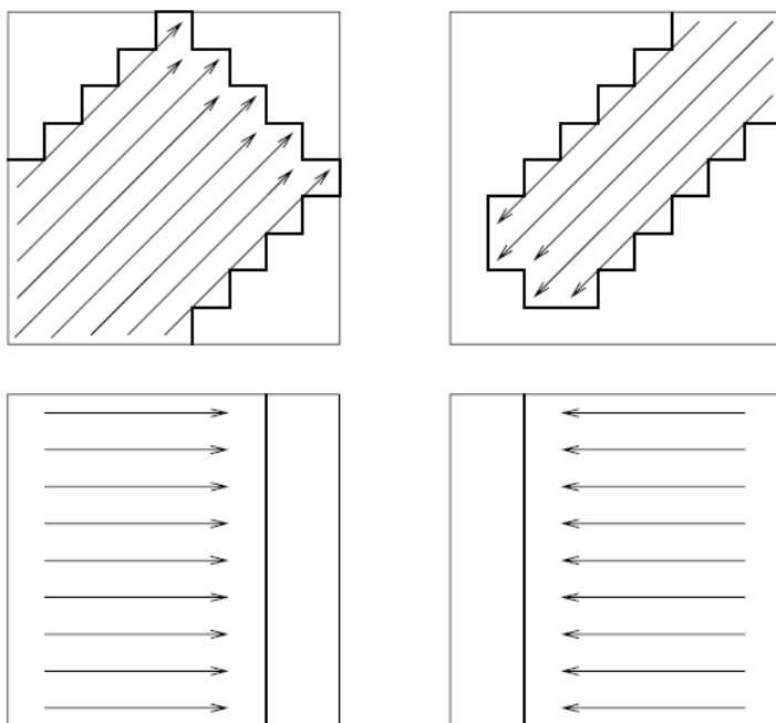
2.6. ábra. Erdős-Selfridge tétel alkalmazása a 13-amórára [4]
