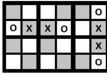
4.9. ábra. 4-sütik blokkolják a két irányú 3-amóbát
