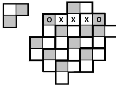
4.10. ábra. 3-sütik blokkolják a két irányú 4-amóbát
